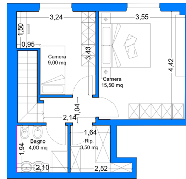
PIANO PRIMO
