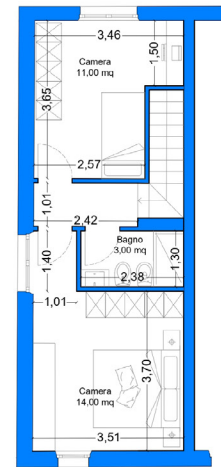
PIANO PRIMO
